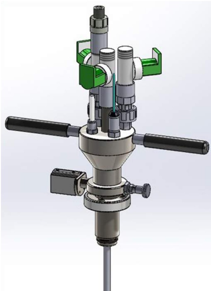
Rendering valvola multipla macchina da caffè
