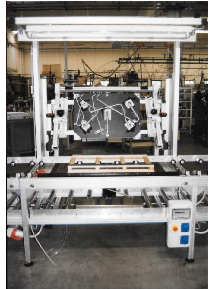
Maschera per montaggio rampe gas
